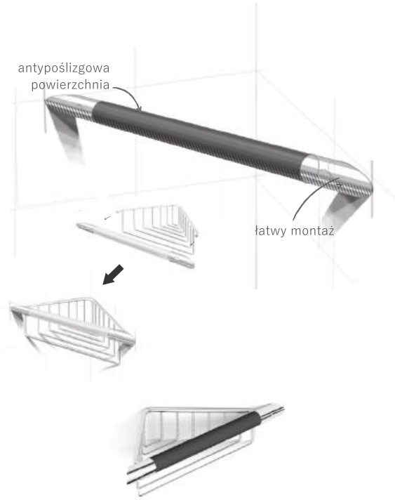
Koszyk narożny z uchwytem 16.039-B Chrom, antypoślizgowy uchwyt w kolorze czarnym 24 x 24 x 7 cm
